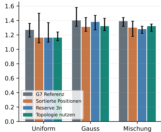
Gesamtprozess [s]
