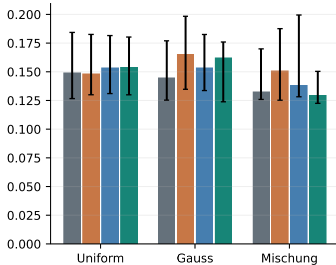
Kraftbaumvorbereitung [s]
