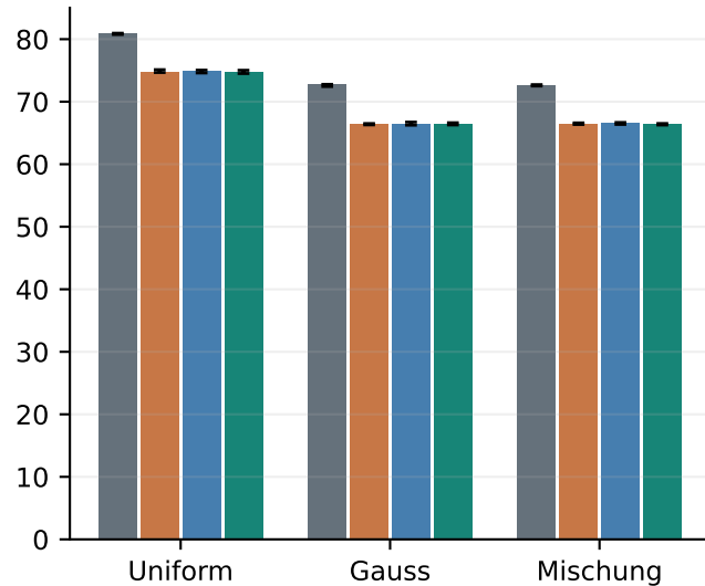
Spitzenspeicher [MiB]
